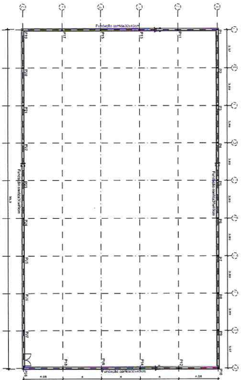
Locação dos Pilares Escala 1:10
